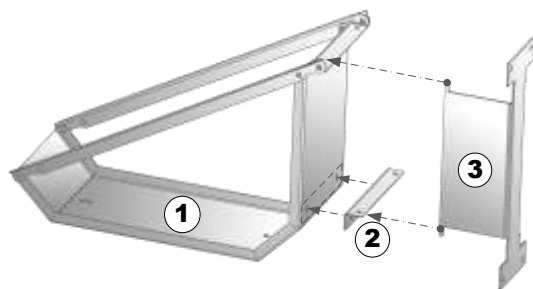
Рис. 1 Кассета рукавная Л01 стандартное исполнение
